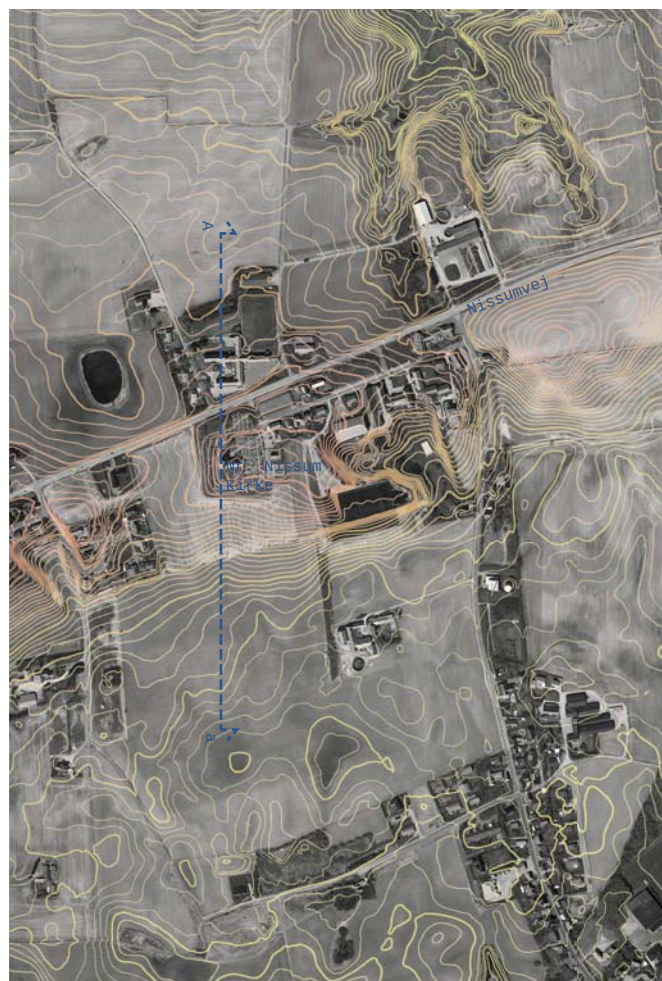
Figur 11 Koteplan med tilhørende principsnit af randmorænen, det forhøjede landskab med Nørre Nissum Kirke.
