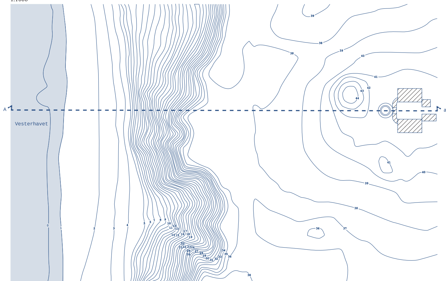
Figur 18 Plan og snit ved Bovbjerg Fyr 1:1000
