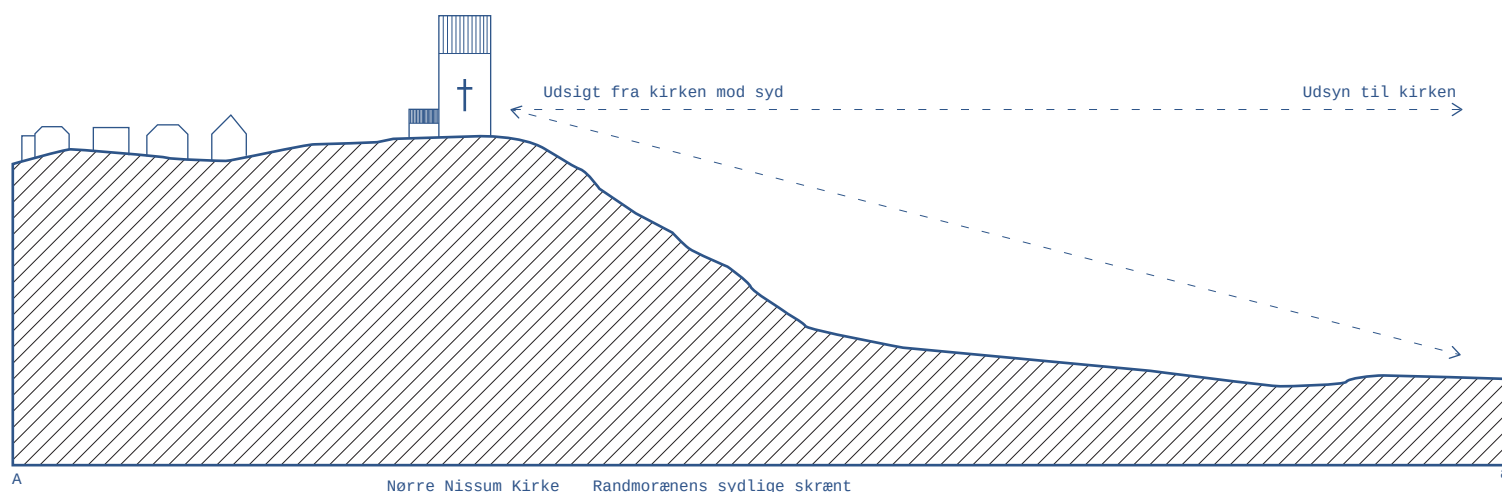
Figur 11 Koteplan med tilhørende principsnit af randmorænen, det forhøjede landskab med Nørre Nissum Kirke.
